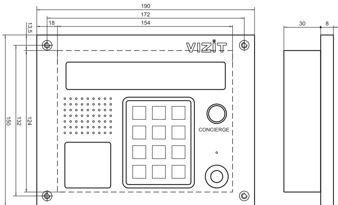
Рисунок 1 - Габаритные и установочные размеры блока вызова БВД-431
