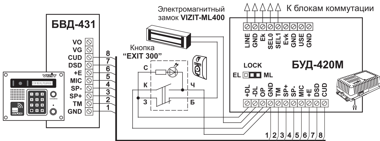
Рисунок 3 - Схема соединений блока вызова БВД-431 с блоком управления БУД-420М , электромагнитным замком VIZIT-ML400 и кнопкой “EXIT 300”
