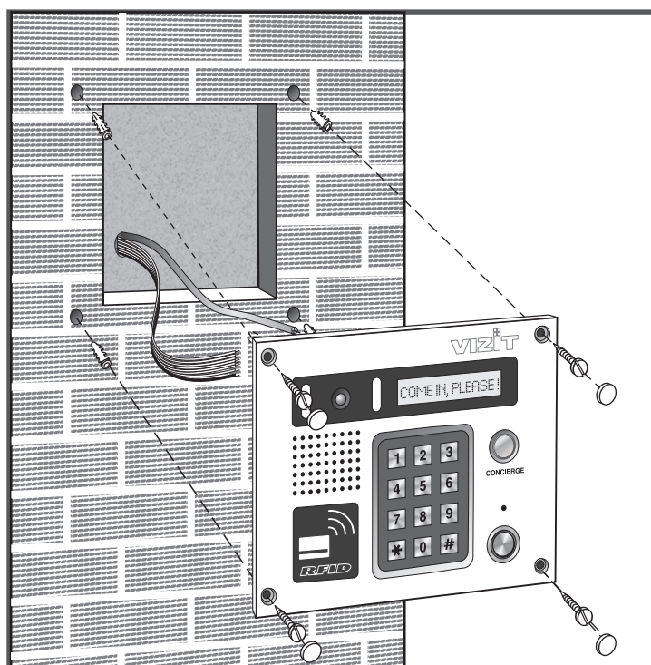
Рисунок 2 - Крепление блока вызова
